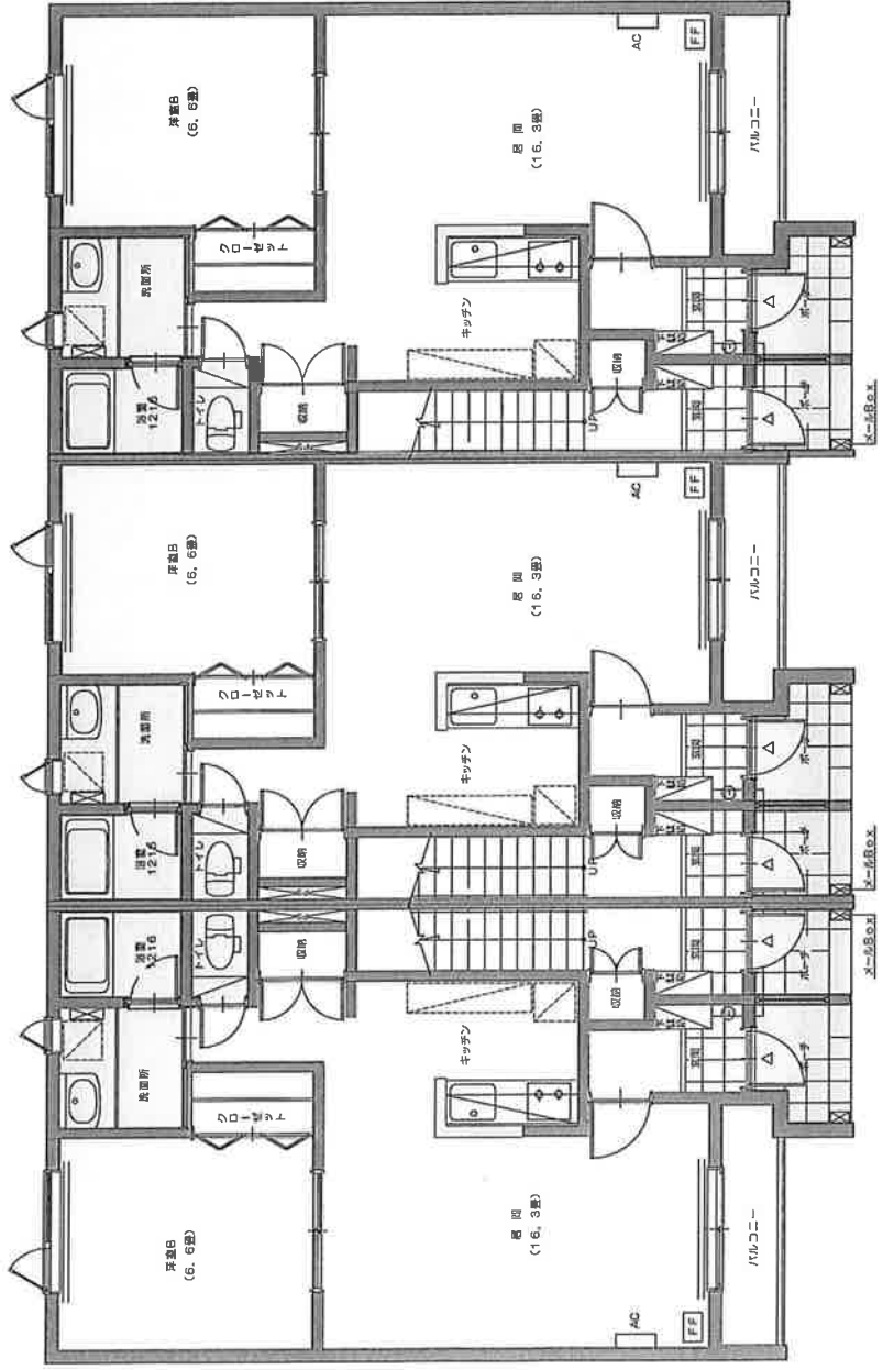
A棟1階平面図
