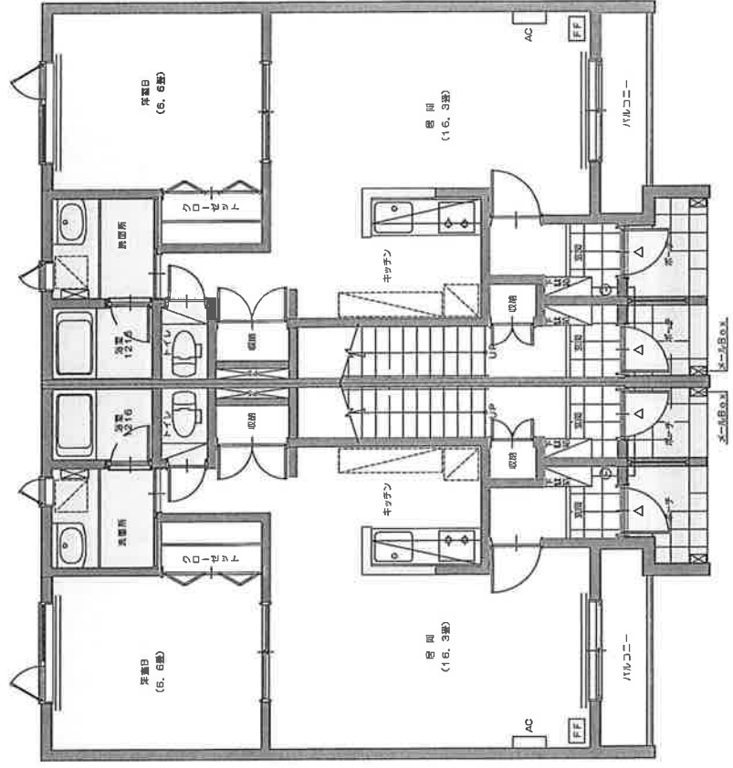
B棟1階平面図
